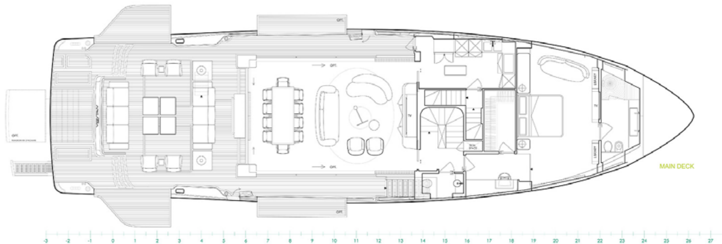
ГЛАВНАЯ ПАЛУБА
