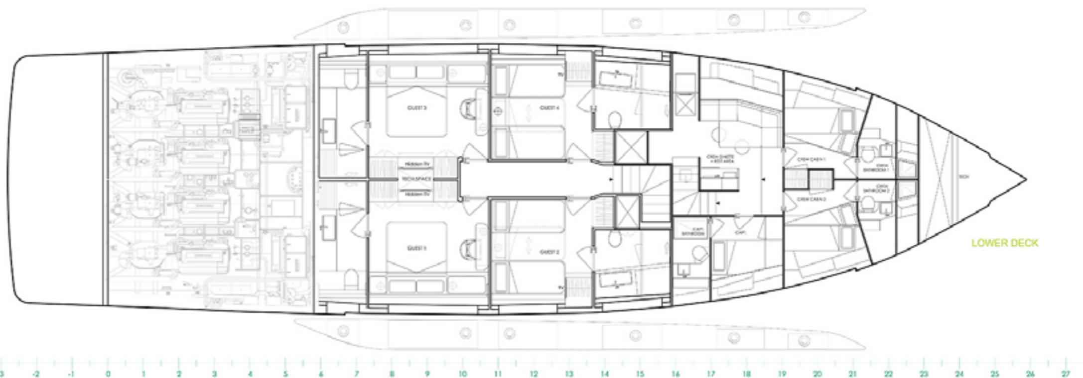
НИЖНЯЯ ПАЛУБА
