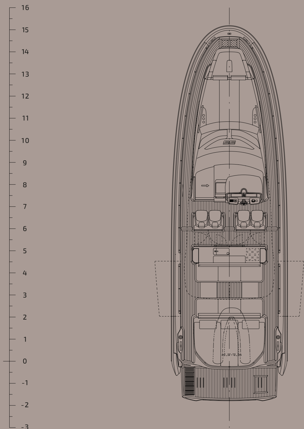
ГЛАВНАЯ ПАЛУБА
