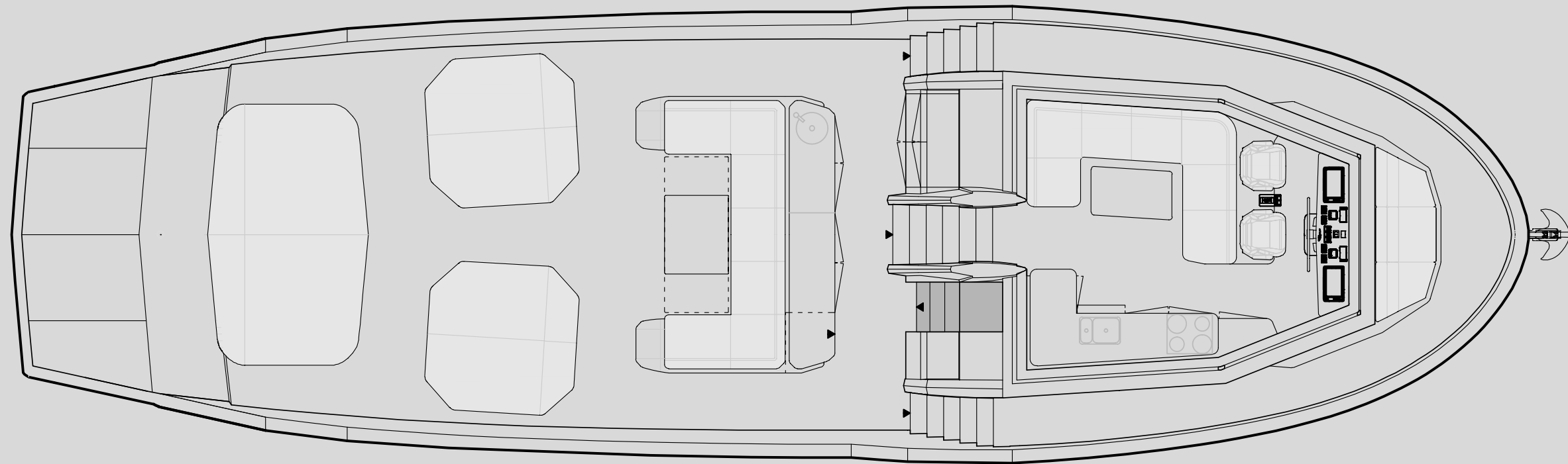
ГЛАВНАЯ ПАЛУБА
