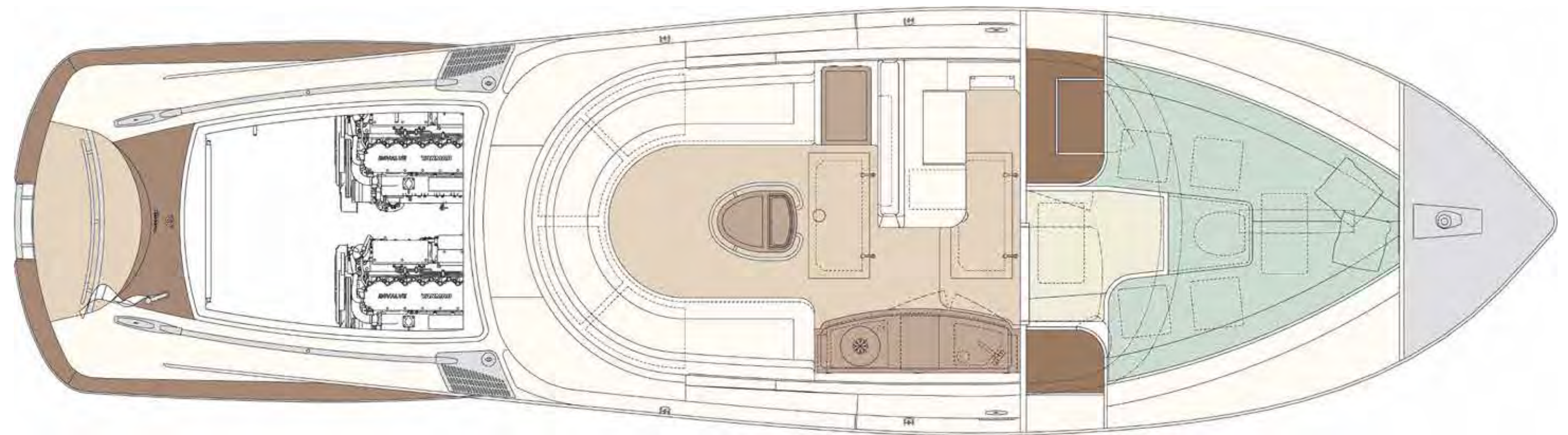
НИЖНЯЯ ПАЛУБА
